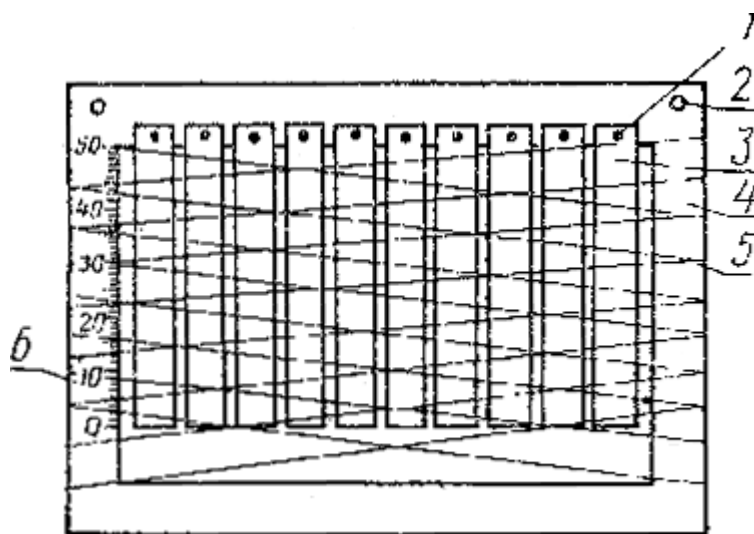
1- игла для крепления образцов; 2- отверстия для крепления рамки в термостате или туннельной печи; 3-испытуемые образцы; 4- рамка; 5- нитки; 6-шкала
